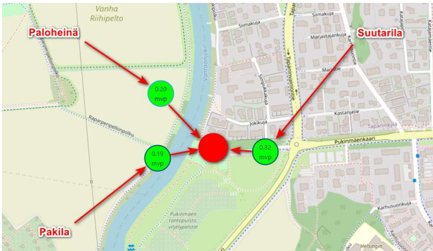
Kuva 2 Pukinmäen pumppaamo keskellä ja isojen viettoviemärien pinnanmittaukset
