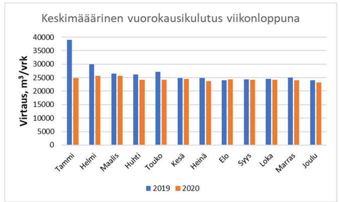
Kuva 65. Halisten haaran mitatut keskimääräiset kuukausittaiset vuorokausikulutukset arkipäiville ja viikonloppulle vuosina 2019 – 2020.
