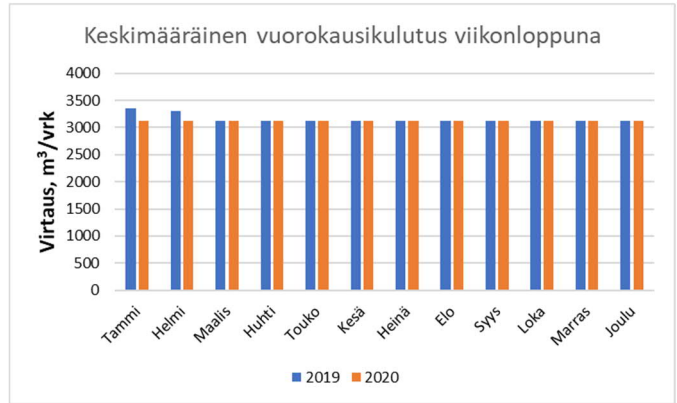
Kuva 64. Moision haaran mitatut keskimääräiset kuukausittaiset vuorokausikulutukset arkipäiville ja viikonloppulle vuosina 2019 – 2020.
